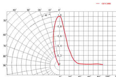
Исполнение «Г30»
