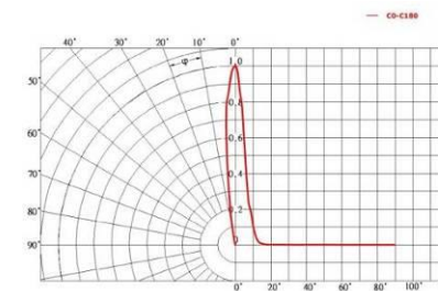
Исполнение «Г60»
