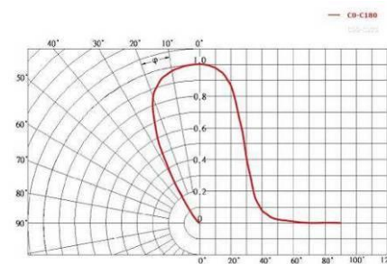
Рисунок 4 Типы КСС
